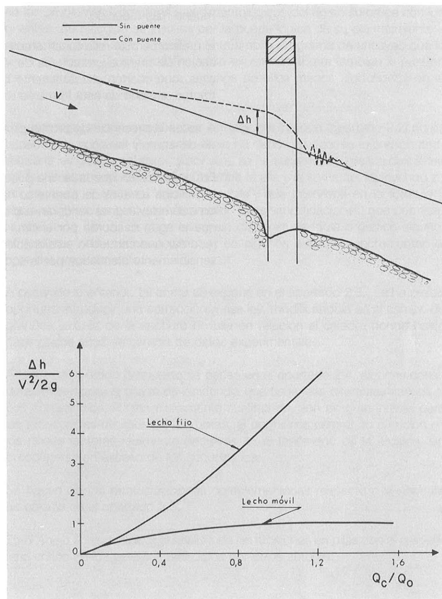
Fig. 1.5. REMANSO PRODUCIDO POR LA PRESENCIA DE PUENTES EN EL CAUCE DEL RIO
