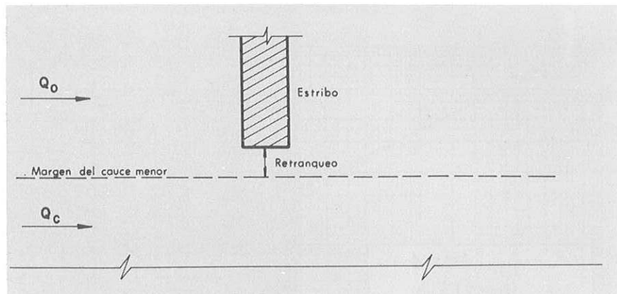
Fig. 3.2. ESTRIBO RETRANQUEADO SITUADO EN CAUCE DE AVENIDAS
