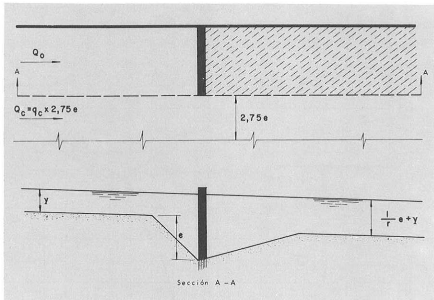
Fig. B.2. ESQUEMA DE DEFINICION DE UN ESTRIBO LARGO SITUADO EN EL CAUCE DE AVENIDAS
