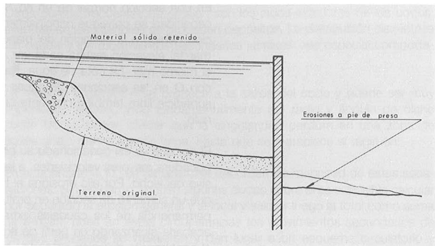
Fig. 4.6. ALTERACION DEL LECHO DEL RIO DEBIDO A LA EXISTENCIA DE UN EMBALSE
