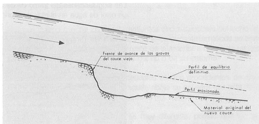
Fig. 4.3. ETAPA DE TRANSICION DEL NUEVO CAUCE
