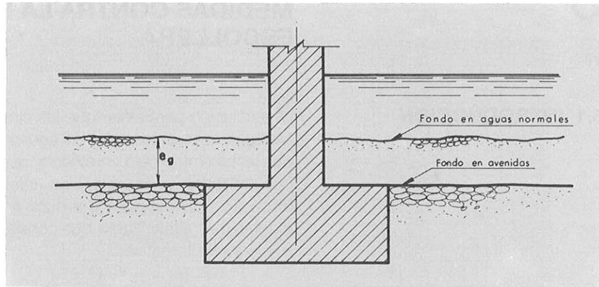
Fig. 5.2. COTA RECOMENDABLE DEL CIMIENTO Y DE LOS MANTOS DE ESCOLLERA
