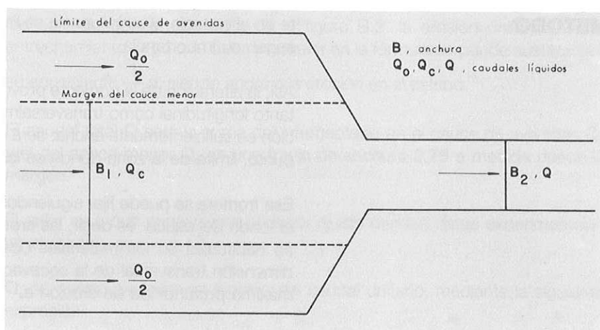
Fig. B.1. ESQUEMA DE DEFINICION DE UN ESTRECHAMIENTO LARGO
