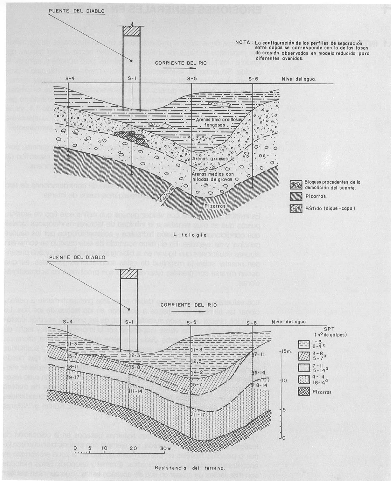
Fig. 4.1. PERFIL LONGITUDINAL DEL RIO LLOBREGAT EN EL PUENTE DEL DIABLO (MARTORELL)
