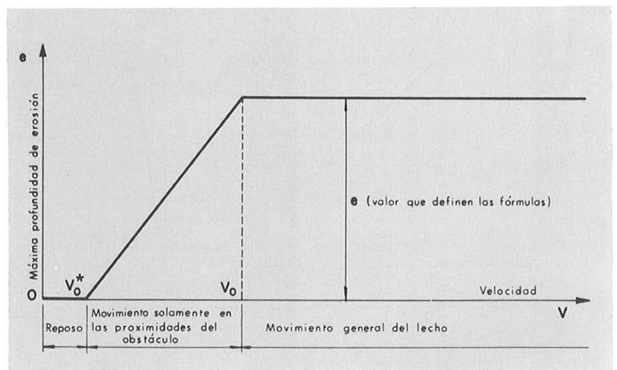
Fig. 1.2. MECANISMO DE DEFINICION DE LA EROSION LOCAL
