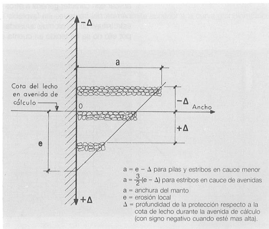
Fig. 5.4. VARIACION DE LA ANCHURA DE LA PROTECCION CON LA COTA
