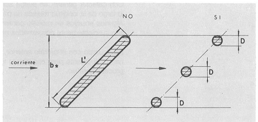
Fig. 2.3. VENTAJAS DEL APOYO MÚLTIPLE CON GRANDES ÁNGULOS DE ATAQUE Y LONGITUDES DE PILA
