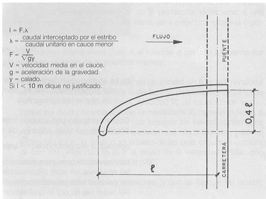
Fig. 5.10. PLANTA DE DIQUE GUIA
