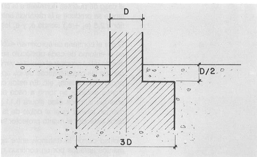
Fig. 5.9. PROTECCION RIGIDA DE CHABERT
