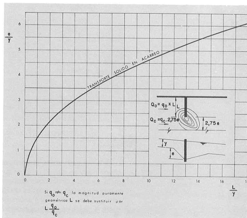
Fig. 3.3. MAXIMA PROFUNDIDAD DE EROSION EN UN ESTRIBO SITUADO SOBRE EL CAUCE MENOR
