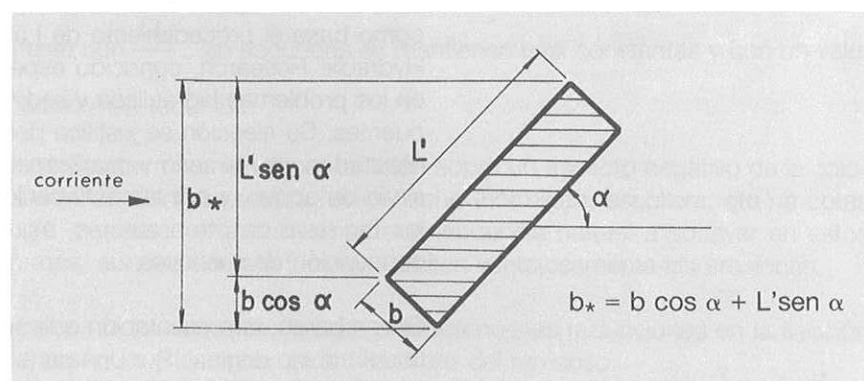
Fig. 2.1. ANCHURA PROYECTADA DE LA PILA
