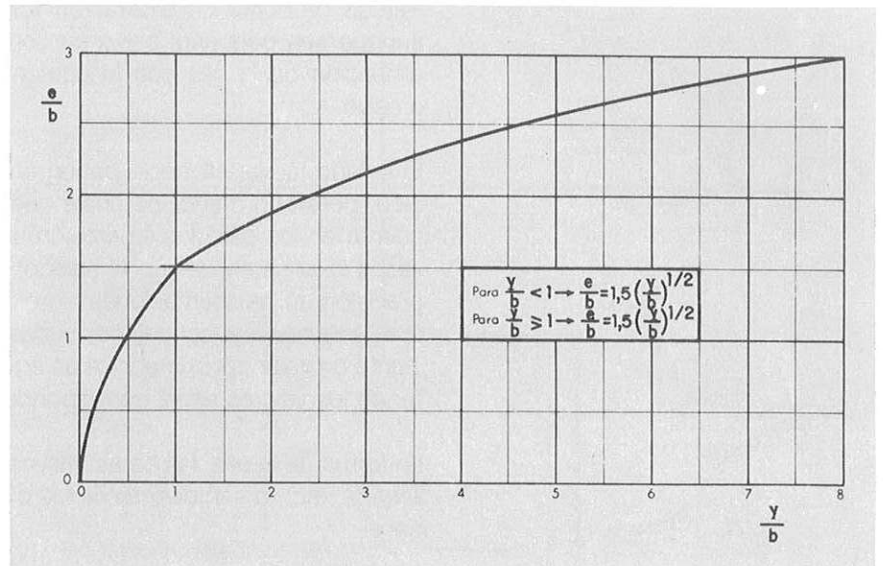
Fig. 2.2. MAXIMA EROSION EN PILAS RECTANGULARES – LEY PROPUESTA
