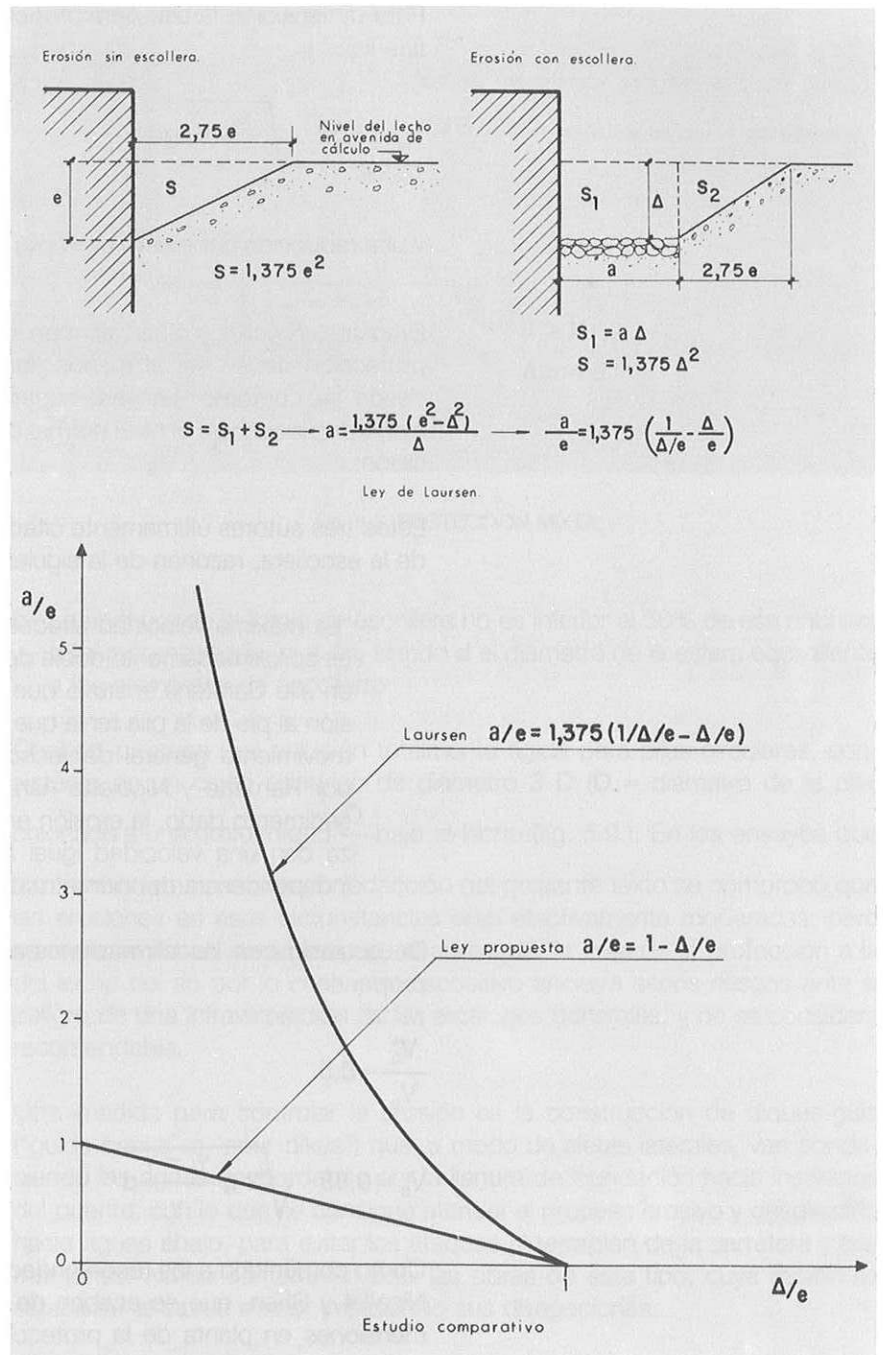
Fig. 5.7. ANCHURA DEL MANTO DE ESCOLLERA SEGUN LAURSEN Y COMPARACION CON LA PROPUESTA EN ESTE TEXTO
