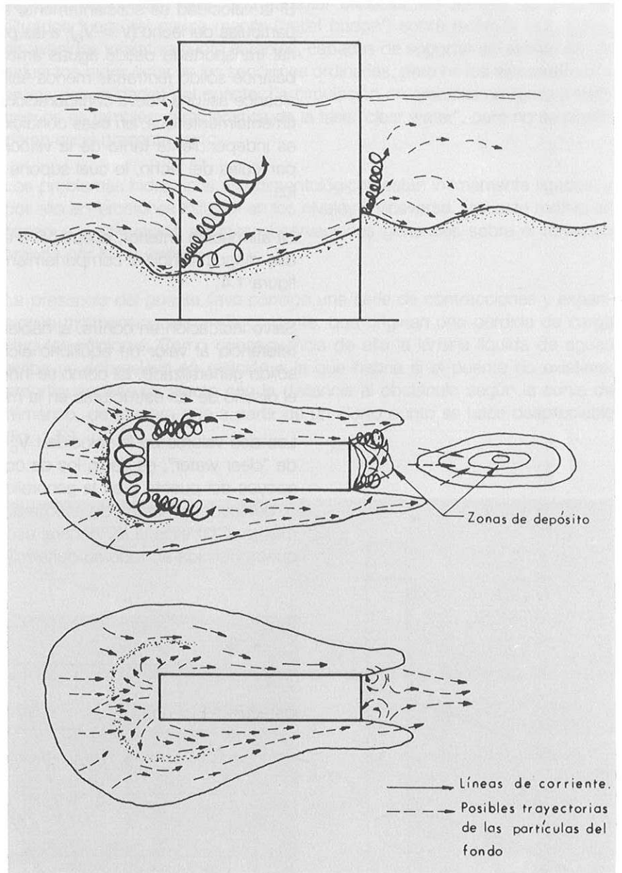
Fig. 1.2. MECANISMO DE DEFINICION DE LA EROSION LOCAL
