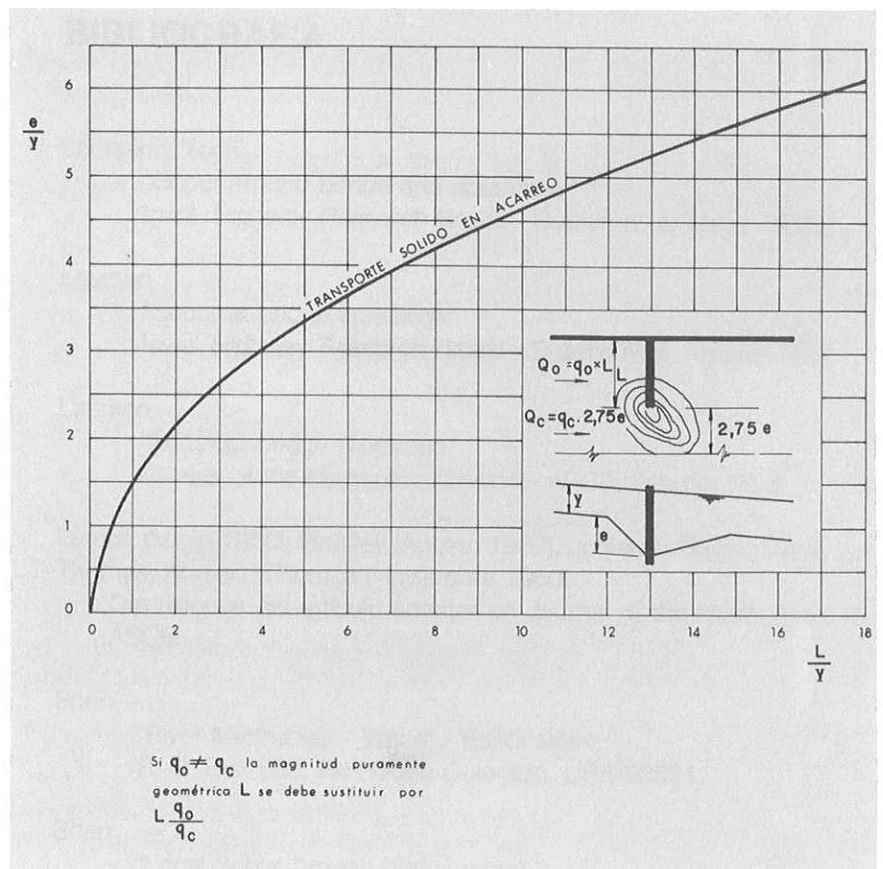
Fig. B.4. MAXIMA PROFUNDIDAD DE EROSION EN UN ESTRIBO SITUADO SOBRE EL CAUCE MENOR
