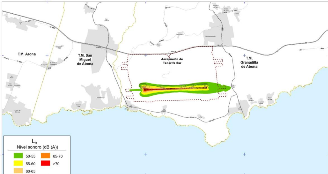
Ilustración 3 Mapa de niveles sonoros Ln. MER Fase IV. Aeropuerto de Tenerife Sur
