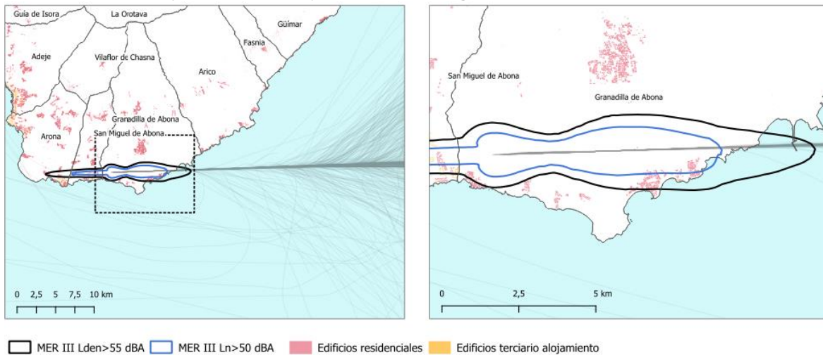
Ilustración 16 Trayectorias aterrizaje habituales configuración Oeste Aeropuerto de Tenerife Sur
