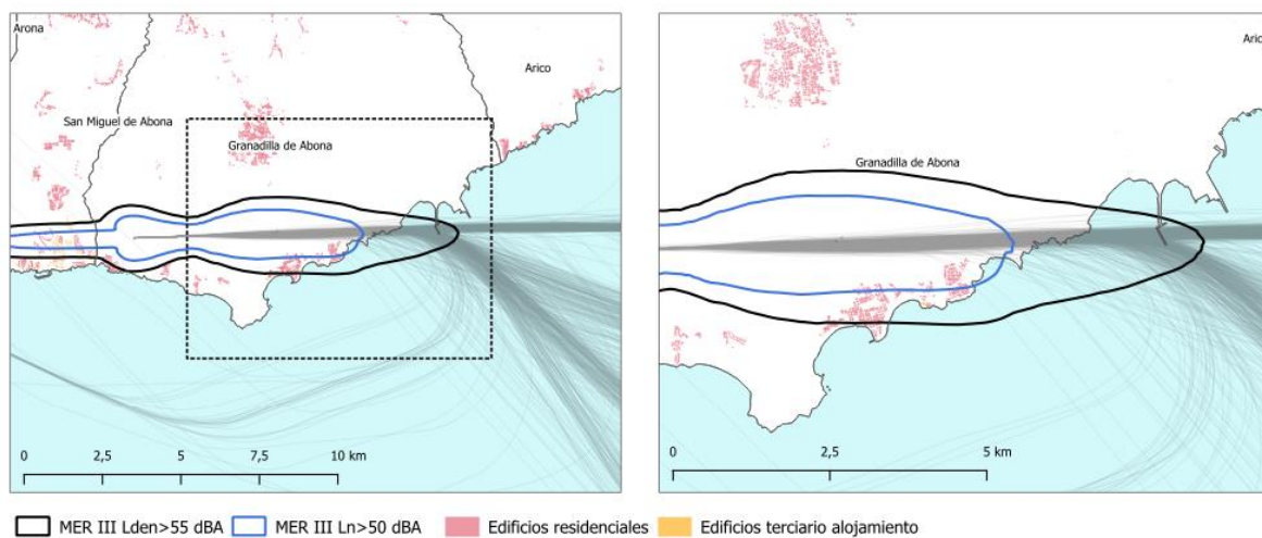
Ilustración 13. Trayectorias despegue habituales configuración Este Aeropuerto de Tenerife Sur
