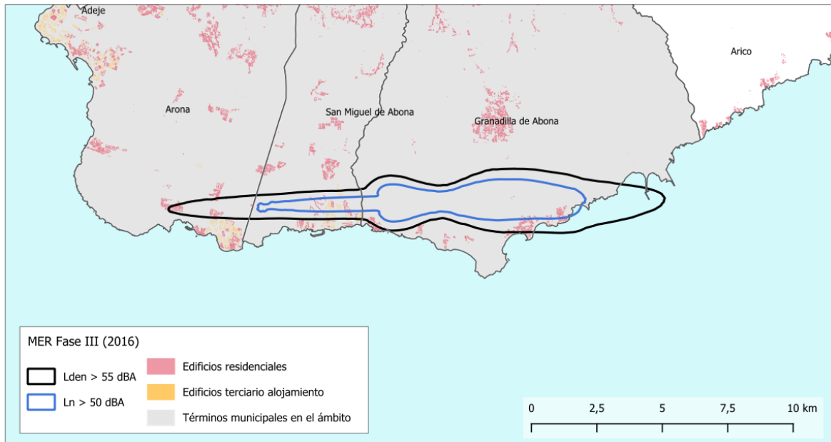
Ilustración 12. Isófonas MER Fase III Aeropuerto de Tenerife Sur
