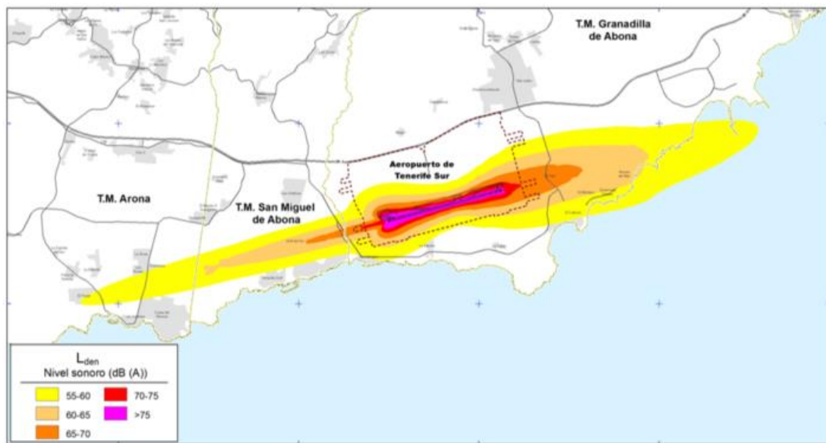
Ilustración 6 Mapa de niveles sonoros L den . MER Fase III. Aeropuerto de Tenerife Sur
