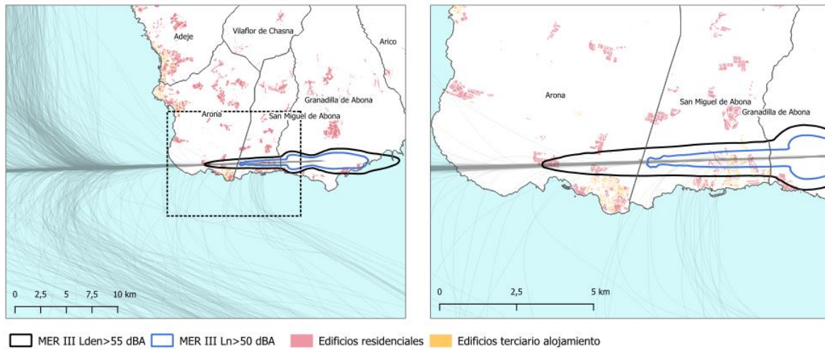
Ilustración 15 Trayectorias aterrizaje habituales configuración Este Aeropuerto de Tenerife Sur
