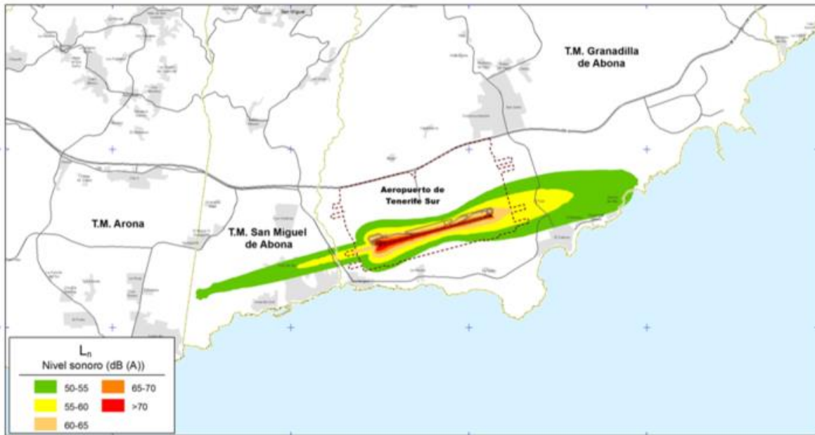
Ilustración 7 Mapa de niveles sonoros L_n . MER Fase III. Aeropuerto de Tenerife Sur
