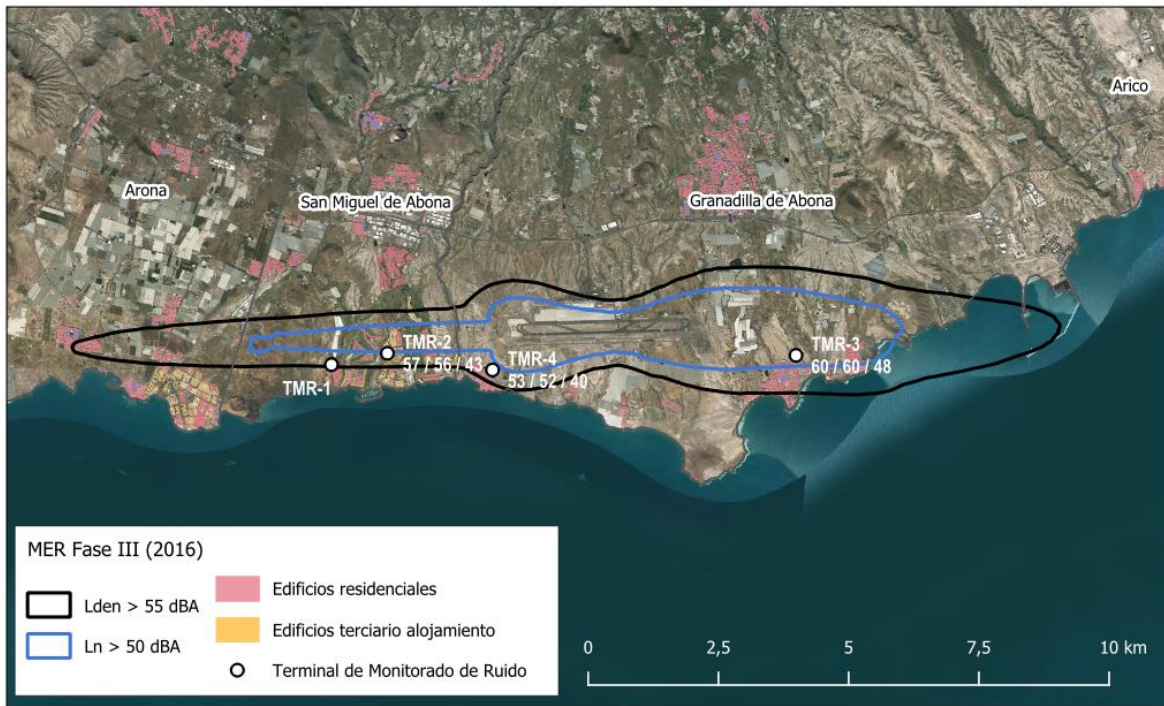
Ilustración 17 Niveles de ruido Laeq avión (D / T / N) del año 2022. Aeropuerto de Tenerife Sur
