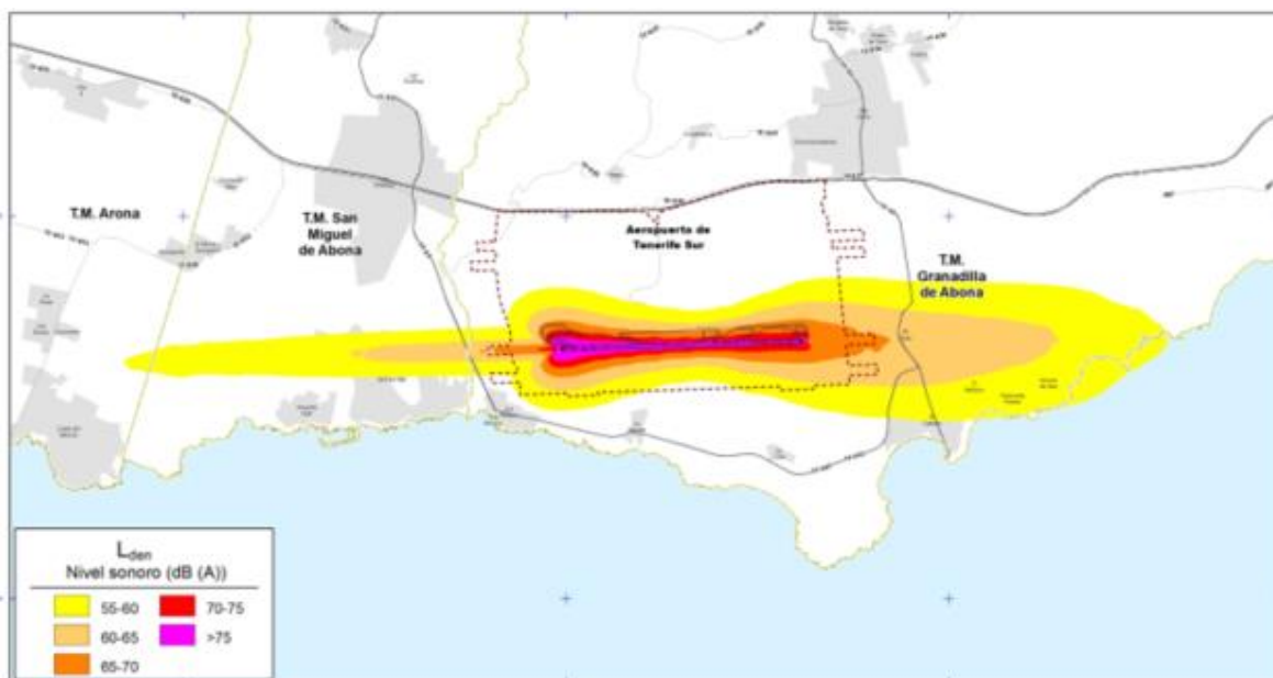
Ilustración 2 Mapa de niveles sonoros L_{den} . MER Fase IV. Aeropuerto de Tenerife Sur
