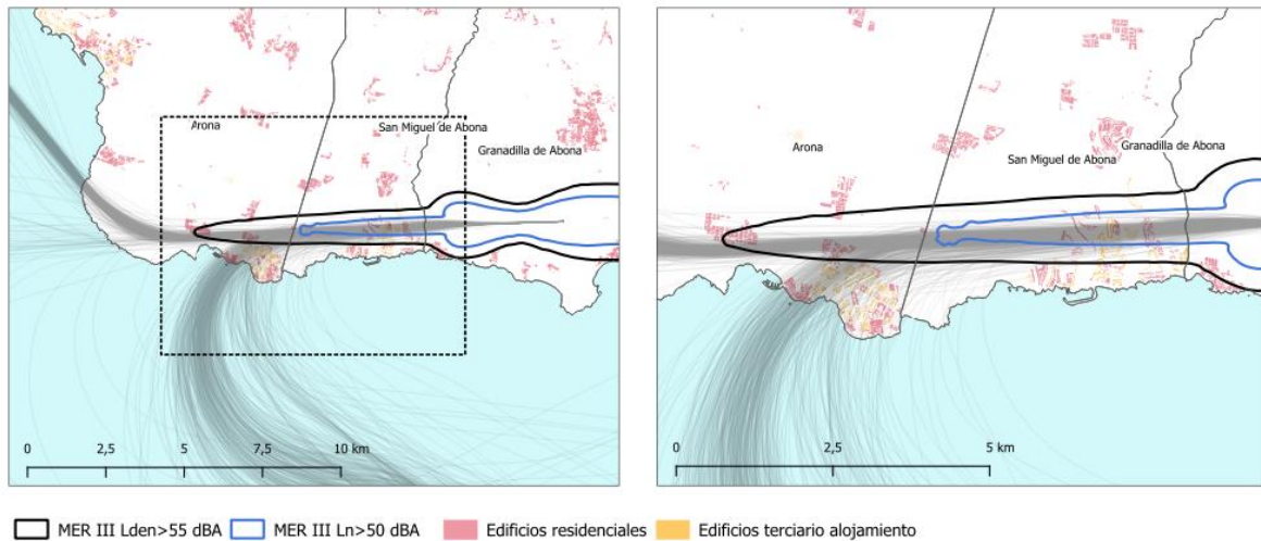
Ilustración 14 Trayectorias despegue habituales configuración Oeste Aeropuerto de Tenerife Sur.
